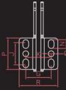
Model: 1102 A
