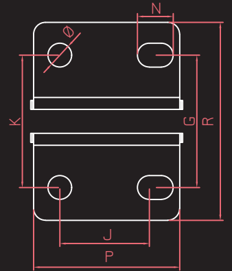
Model: 1104 Y-L
