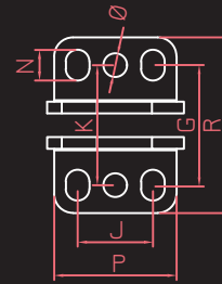
Model: 1101 Y-L
